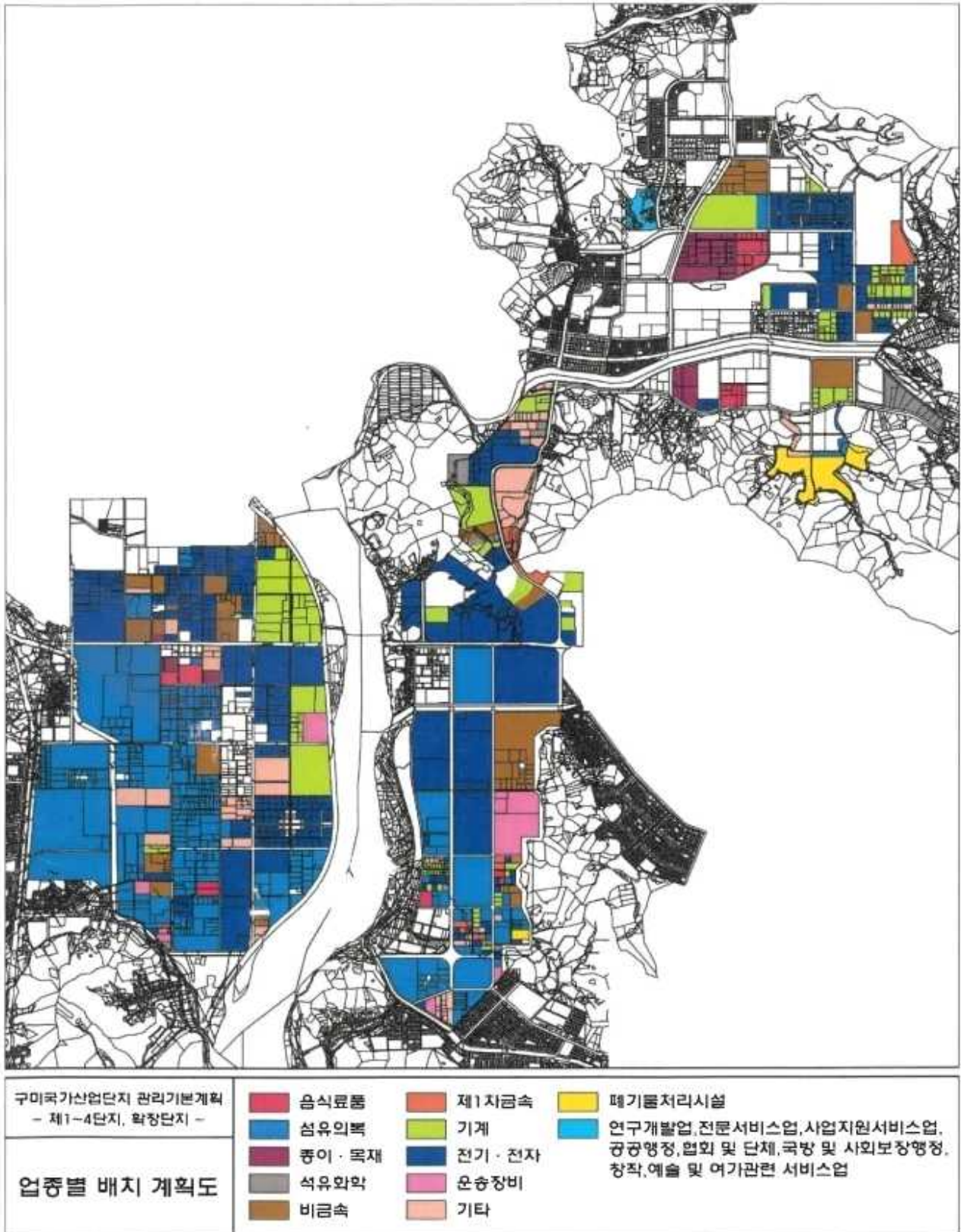
(별첨#3) 구미국가산업단지 업종별 배치도(구미국가 제1~4단지, 확장단지)
